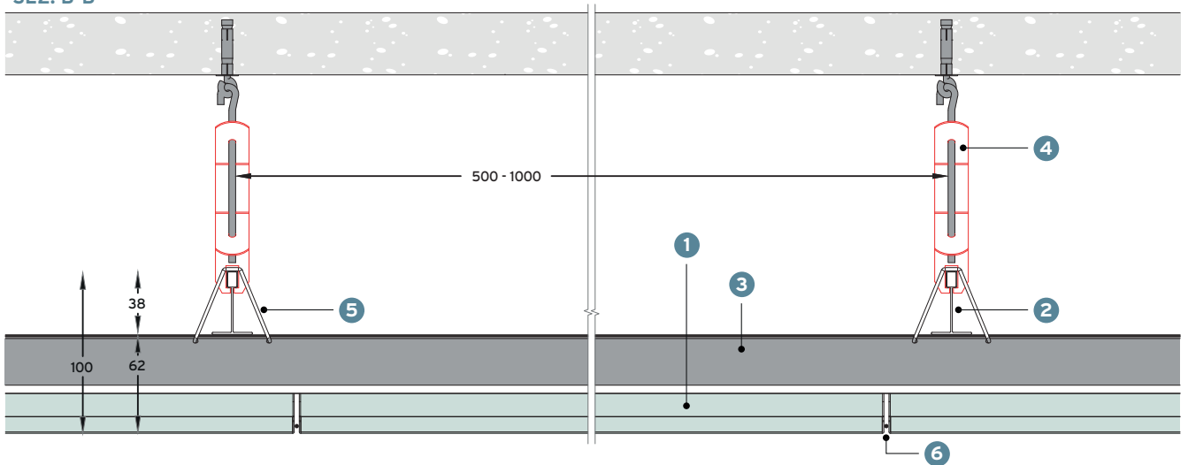
SEZ. B-B
