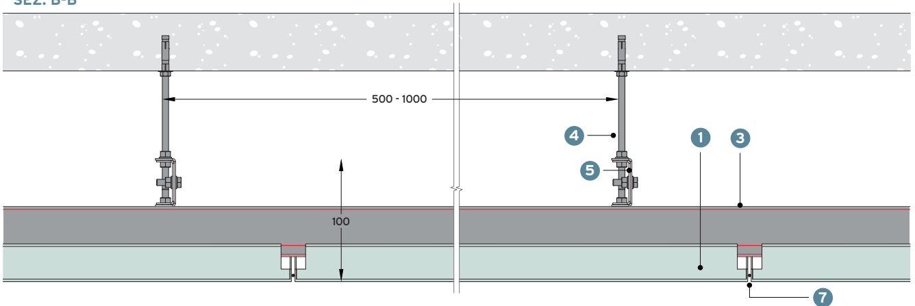
SEZ. B-B
