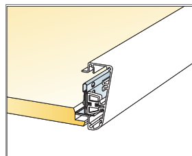
Ühendus plaadid Ds2 poole ja extra profiili vahel
