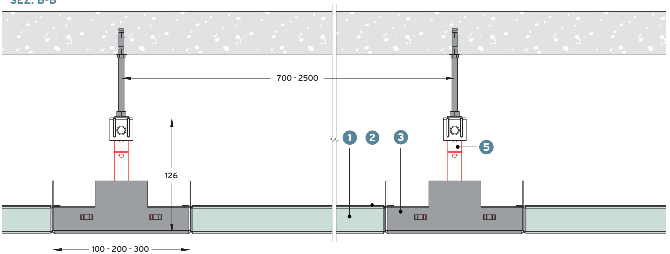
SEZ. B-B
