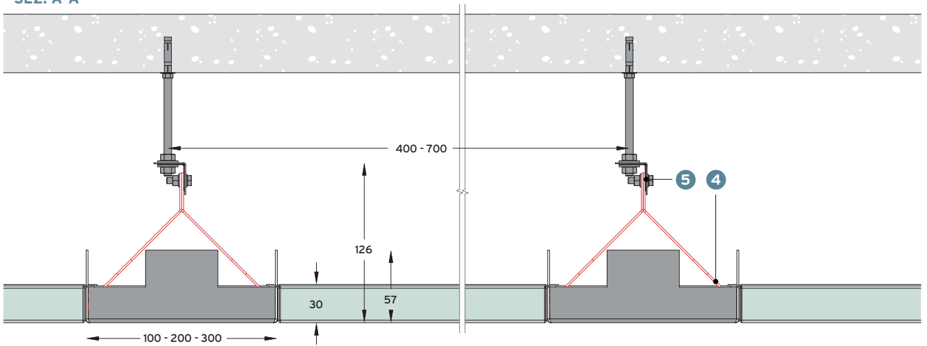
SEZ. A-A
